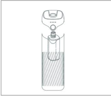
1. הרם את חלקו העליון של המכשיר יש למלא שמן אולטרסוניק בלבד
